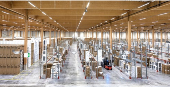
Eligantens lagerhall med limtre fra Moelven Töreboda AB og Moelven Limtre AS.
